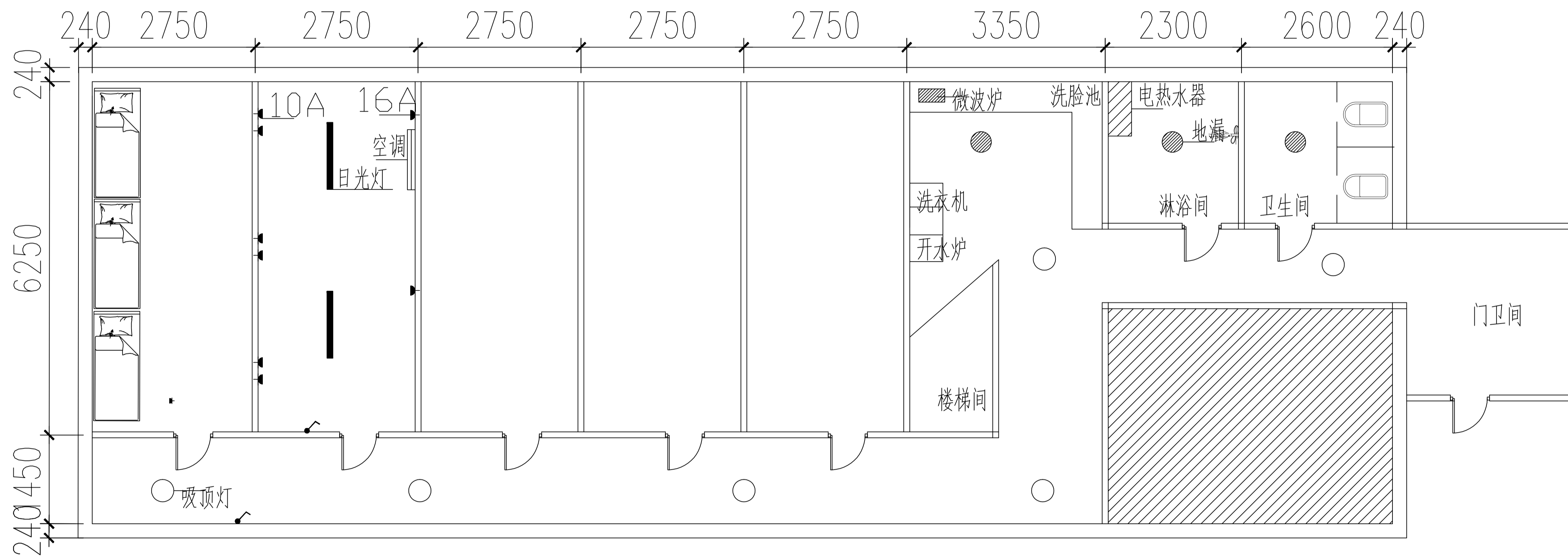
上海生命科学研究院漕宝路园区8号楼车间改造女生宿舍一层平面图
