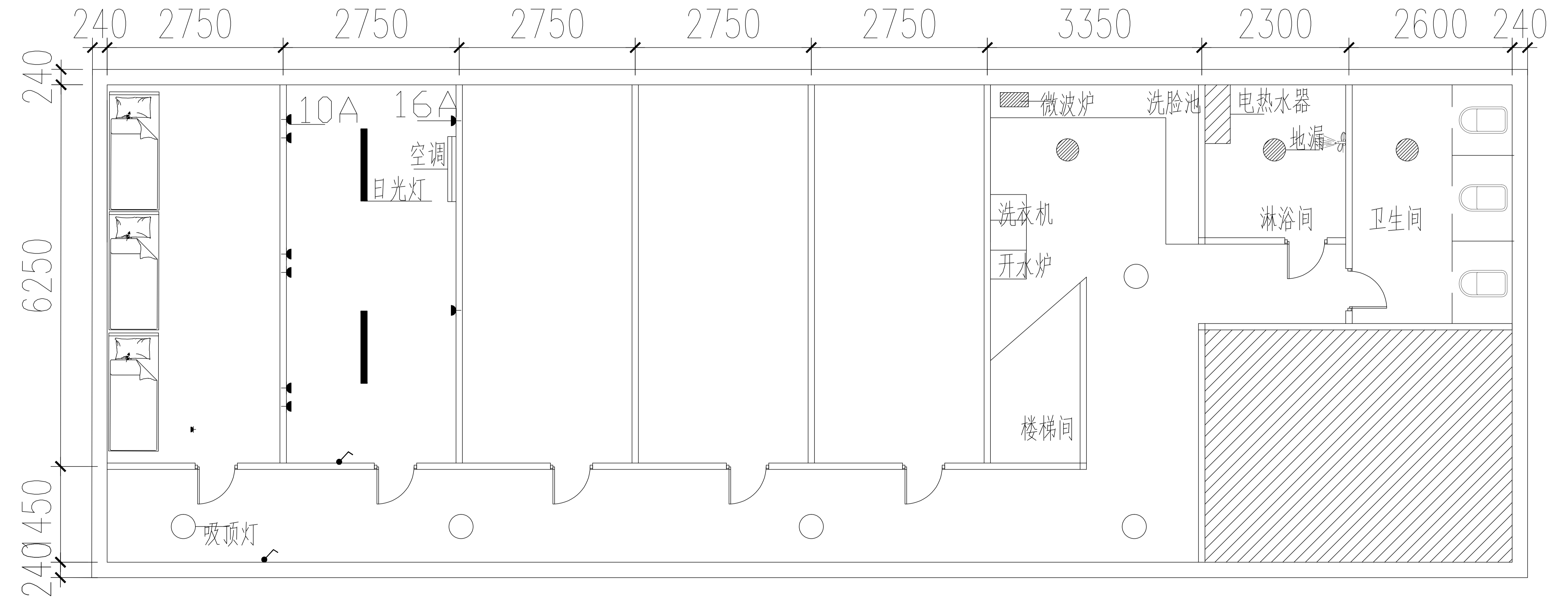
上海生命科学研究院漕宝路园区8号楼车间改造女生宿舍二层平面图
